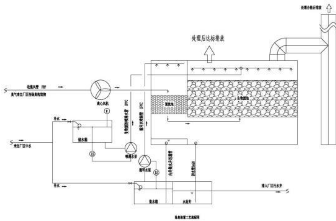
图 4-2 生物滤池除臭工艺流程图
