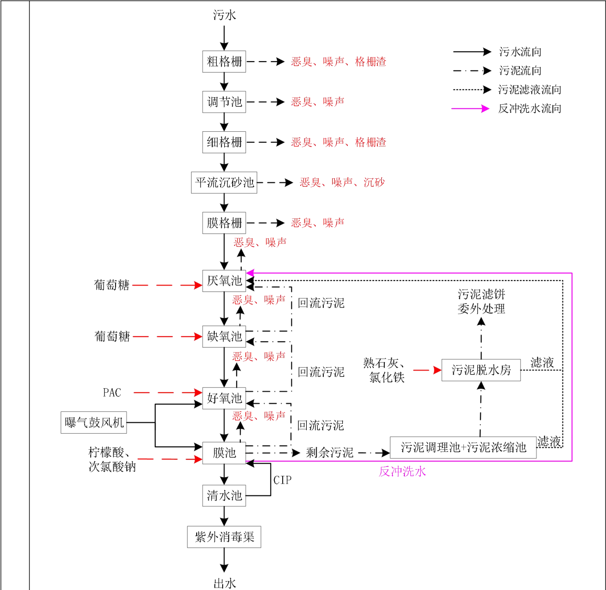
图 4-4 博美镇污水处理厂处理流程图
